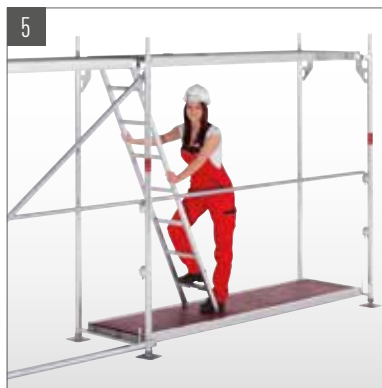
5 Innenliegenden Leitergang auflegen.
