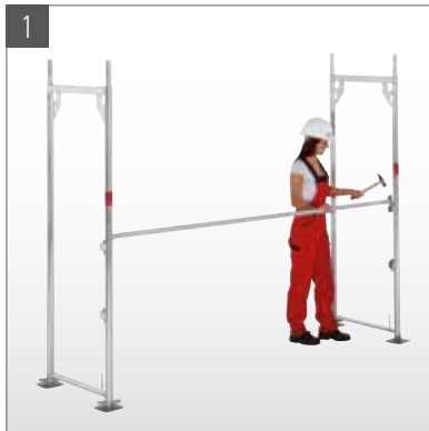
1 Fußspindeln aufstellen, Stellrahmen aufstecken und mit Rückengeländer verbinden.
